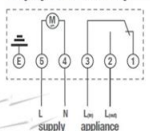
Wiring diagram - Volt Free Switching
